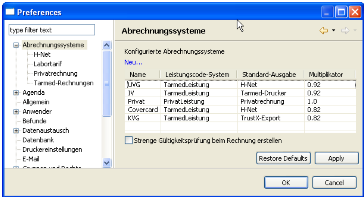
Abbildung 2: Standard-Ausgabeziele festlegen
