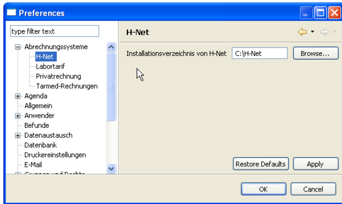
Abbildung 1: Einstellungen H-Net-Client
